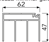
BINARIO SUPERIORE
